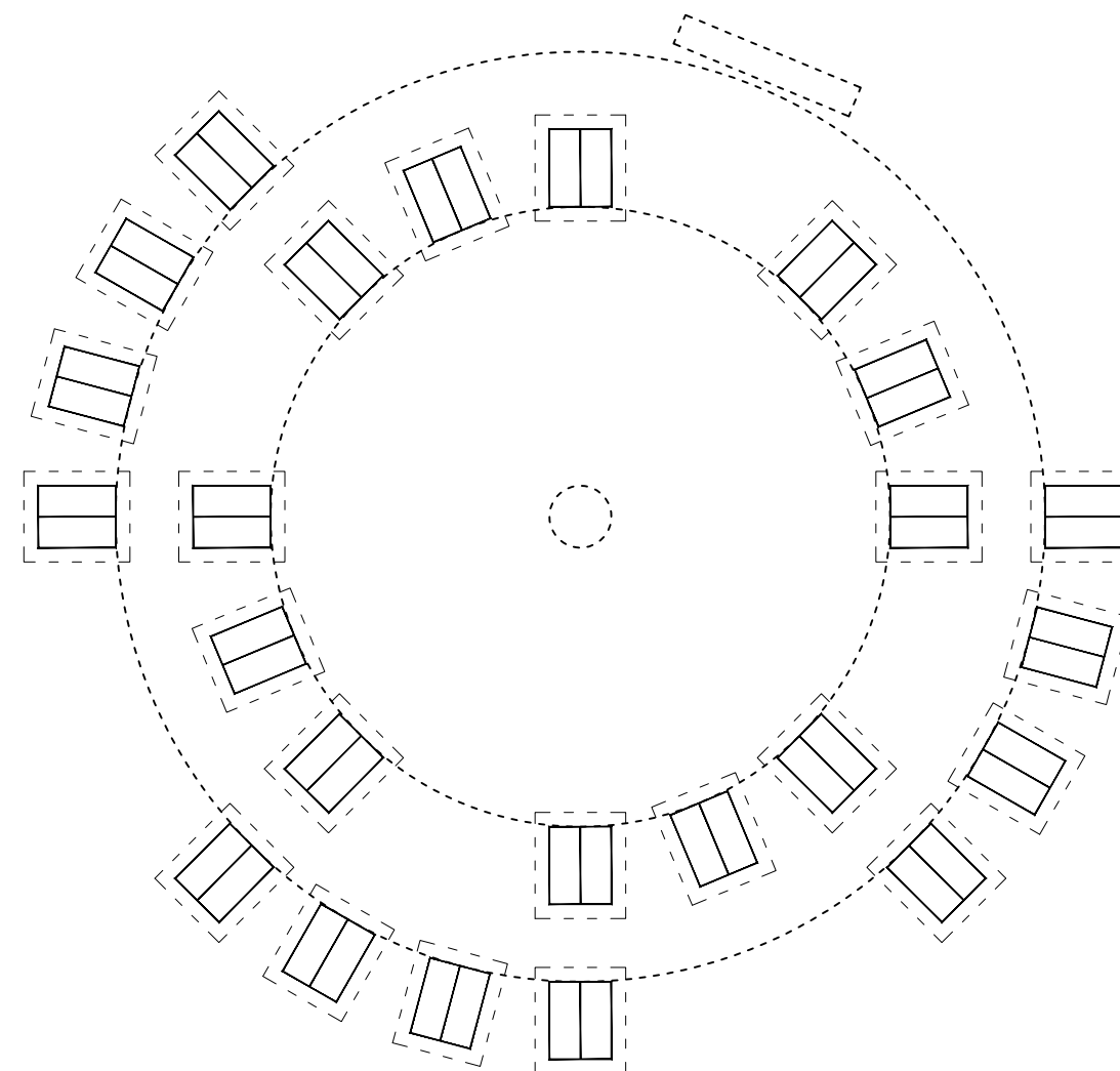
GNIAZDO ok 135 osób 22 (24) namioty - podwójny krąg średnica placu - 40m średnica drugiego kręgu - 60m średnica zewnętrzna - ok 72m
