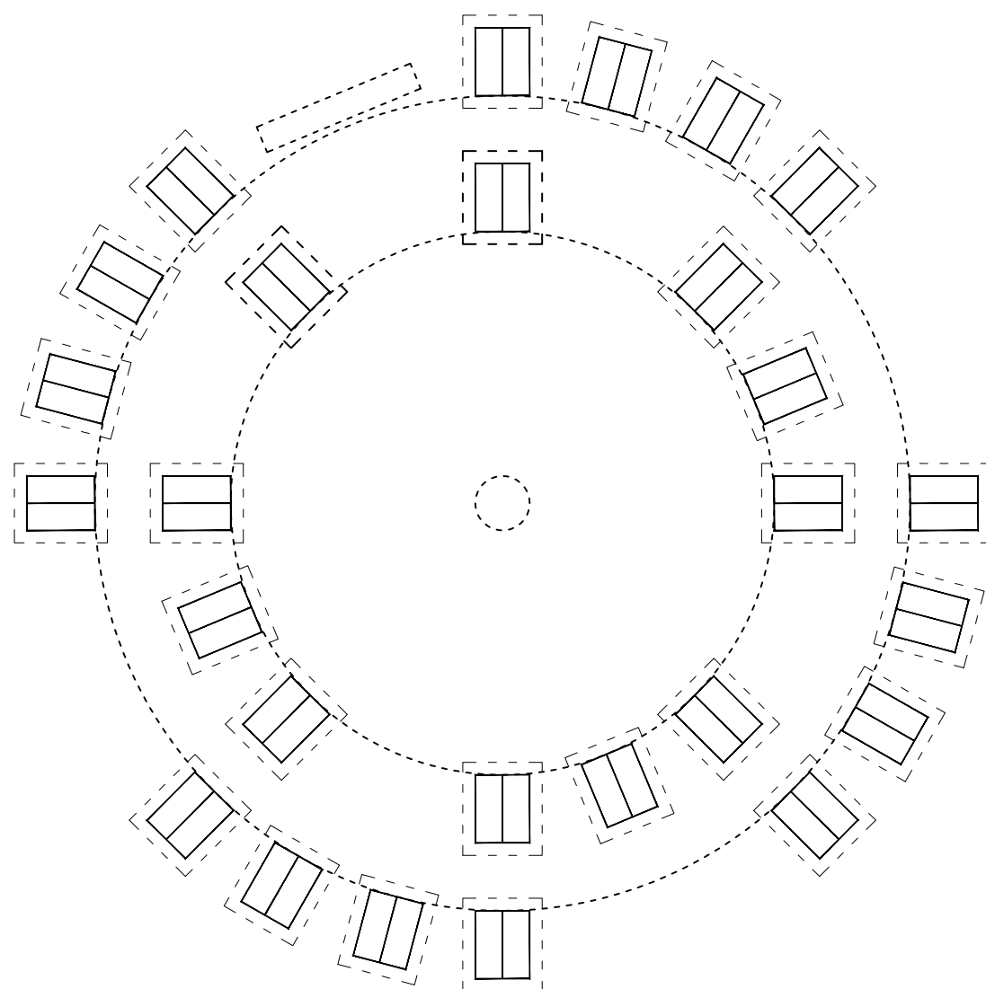
GNIAZDO ok 150 osób 25 (27) namiotów - podwójny krąg średnica placu - 40m średnica drugiego kręgu - 60m średnica zewnętrzna - ok 72m
